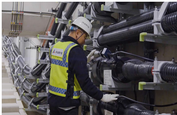
통영천연가스발전사업 건설공사 중 [발전]154kV 송전선로공사 [통영에코파워]
